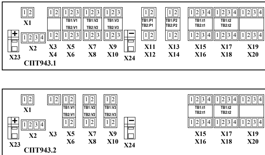
Рисунок 10.1 – Размещение гнезд для подключения внешних цепей
